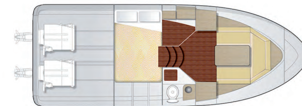
Plan intérieur
